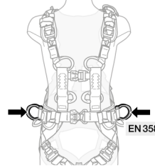
6d. Waistbelt side attachment points Points d'attache latéraux de ceinture
